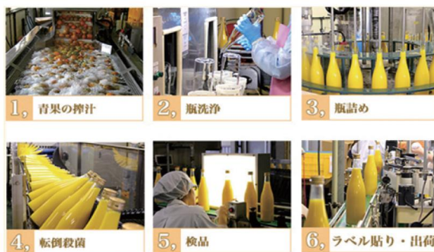
製造工程
