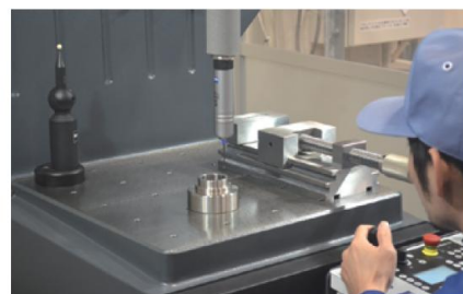
三次元測定器を用いた高精度測定
